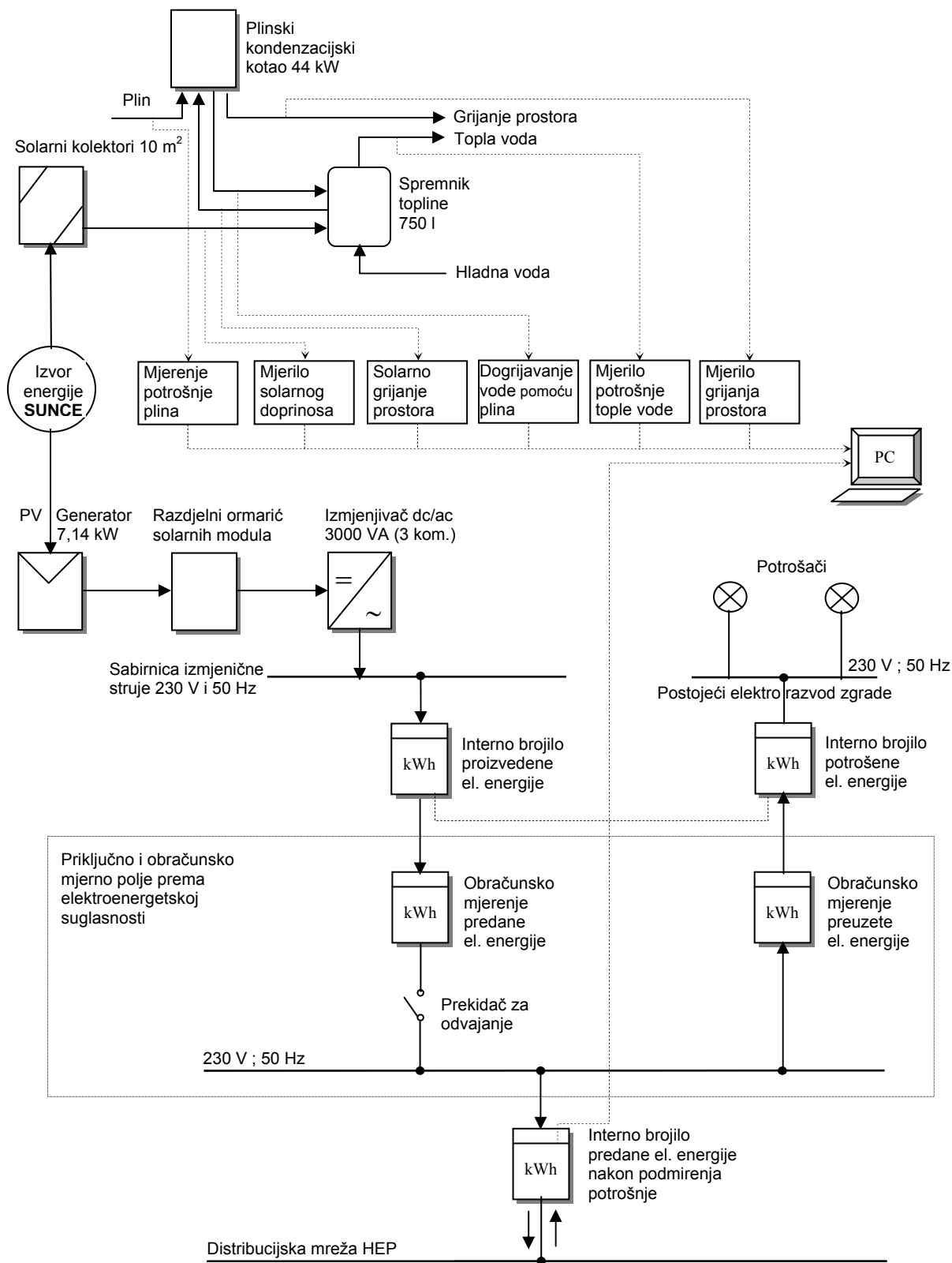
Slika 2. Blok shema proizvodnje toplinske i električne energije projekta “Solarni krov Špansko- Zagreb”
