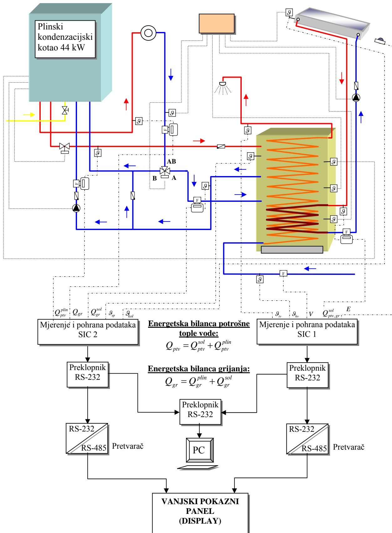
Slika 3. Shema kombinacije plina i solarne energije u sustavu grijanja i pripreme potrošne tople vode na projektu “Solarni krov Špansko-Zagreb”
