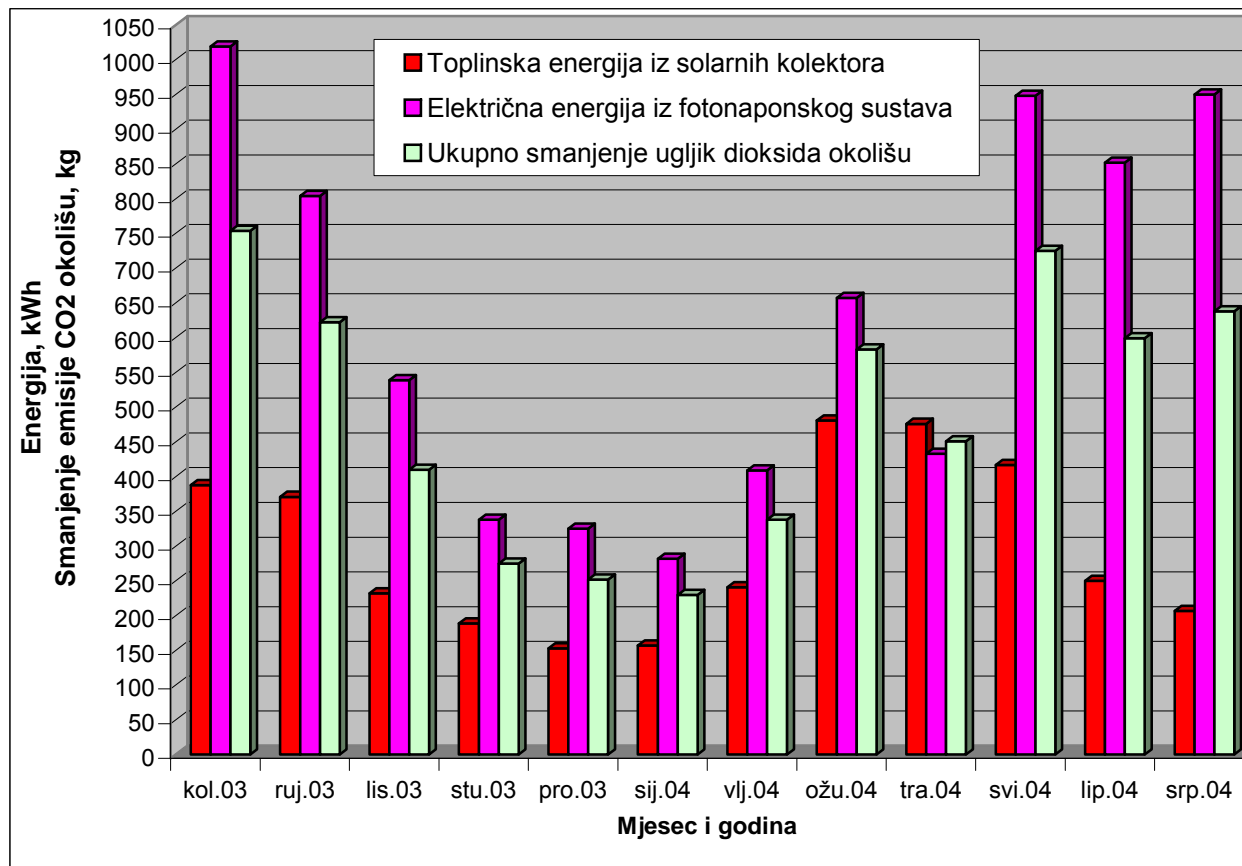
Slika 4. Rezultati mjerenja toplinske i električne energije i smanjenja emisije CO 2 okolišu
